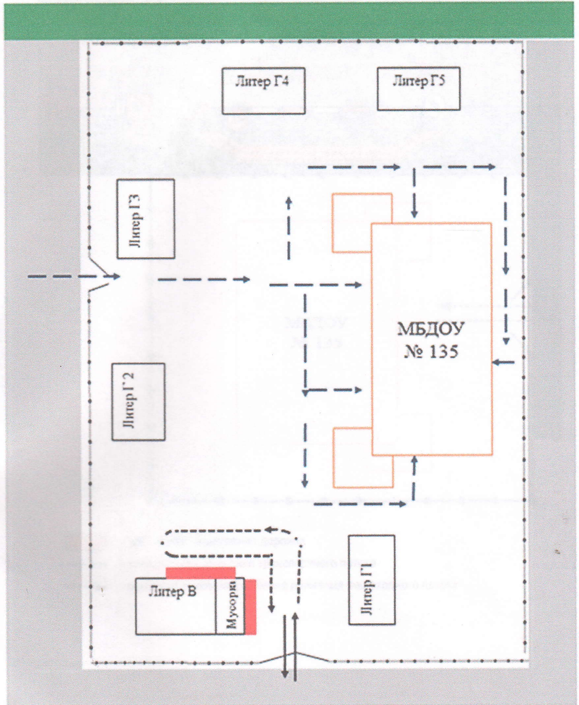
1.3 Схема путей движения транспортных средств к местам разгрузки/погрузки детей по территории МБДОУ МО г. Краснодар «Детский сад № 135»
